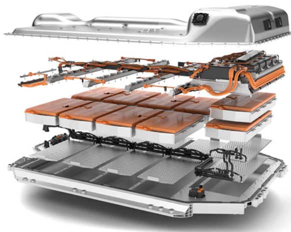
Beispielhafte Darstellung eines Batteriesystems
